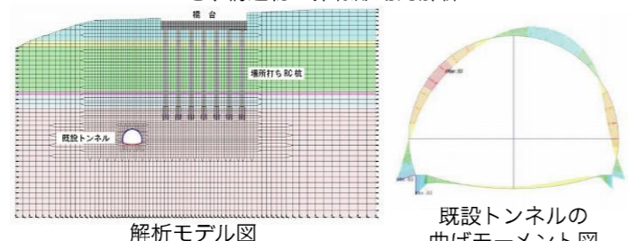
杭施工が既設トンネルに与える影響解析
