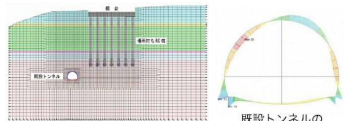
解析モデル図
