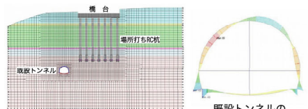
解析モデル図
