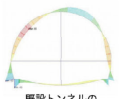
既設トンネルの 曲げモーメント図
