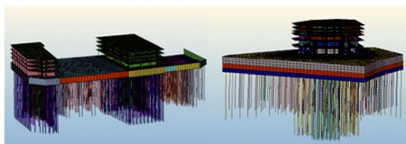
ドバイタワー基礎の解析
