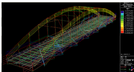
ランガートラス橋の応力解析
